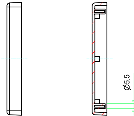
E-E ( 1 : 2.5 )
