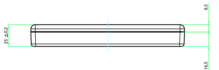
B-B ( 1 : 2.5 )
