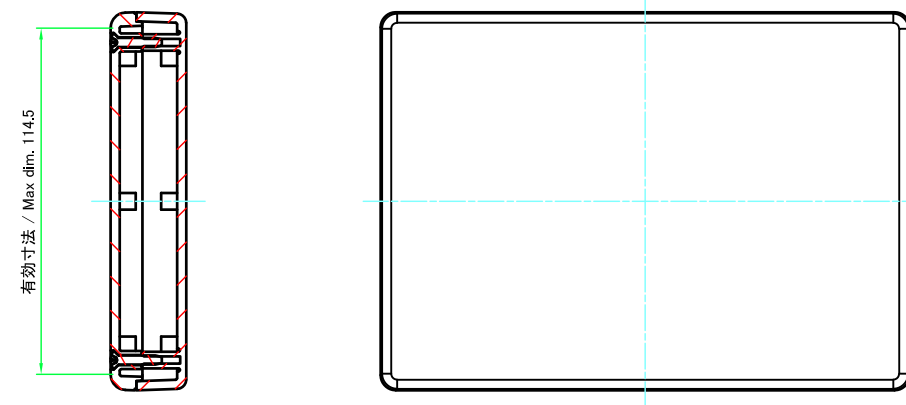
A-A ( 1 : 2.5 )
