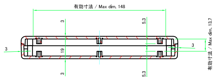
B-B ( 1 : 2.5 )
